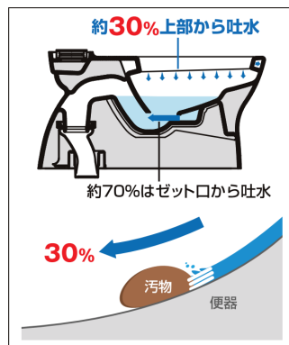
従来型ゼット口付便器
